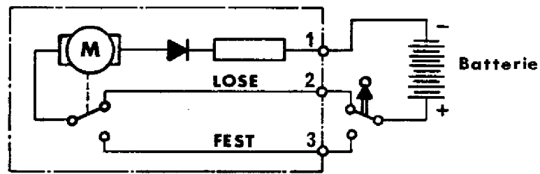
Anschlußschema für Handbremsanzeige:
